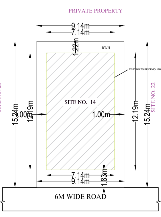
SITE PLAN 1:200
